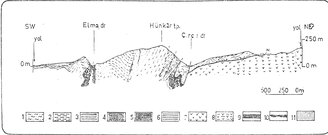
Şek 3 -- istanbul boğazı kuzey kesiminin jeolojik kesitli
